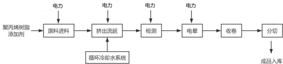
CPP膜生产工艺流程
